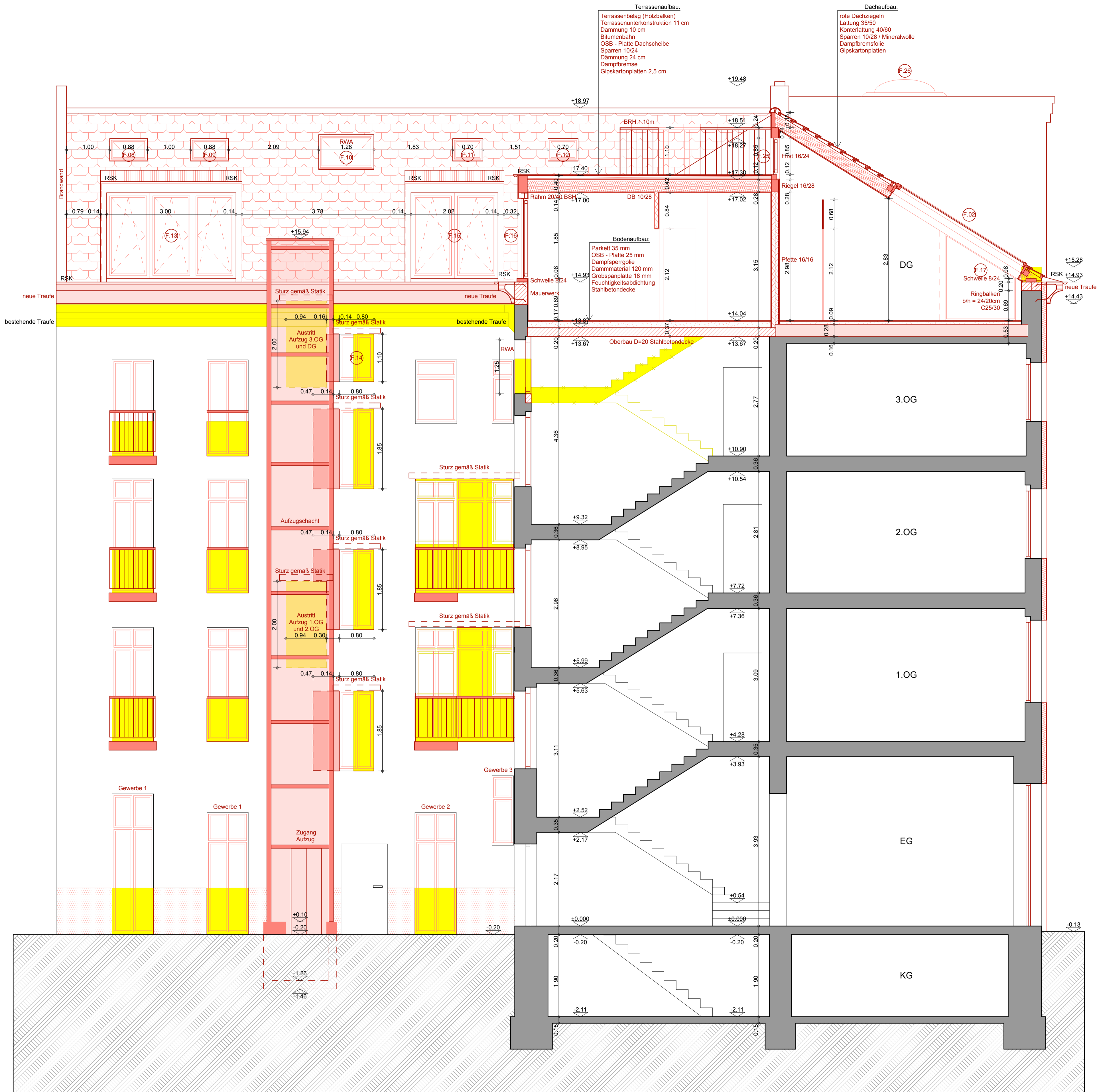
Schnitt B-B
