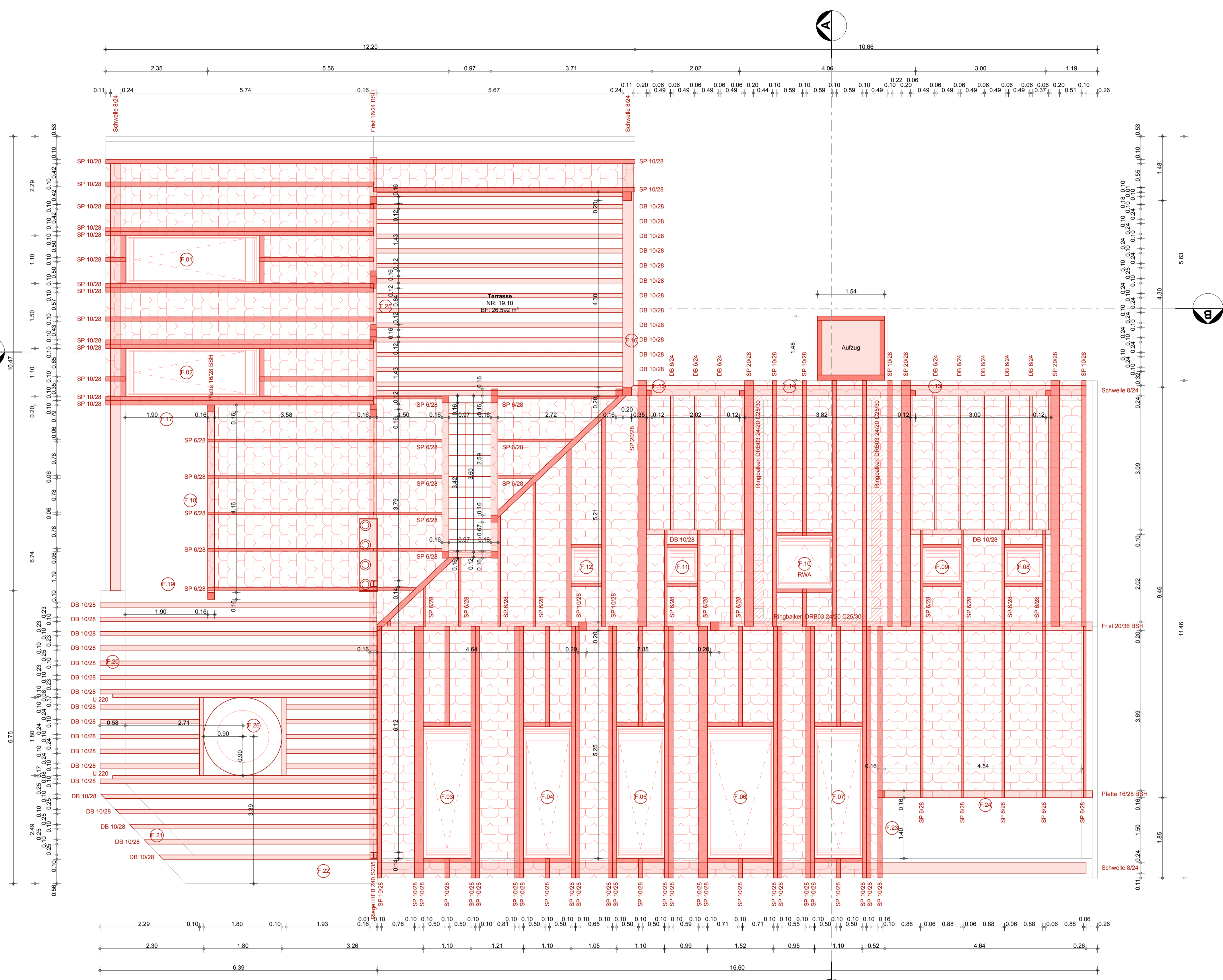
Dachaufsicht
